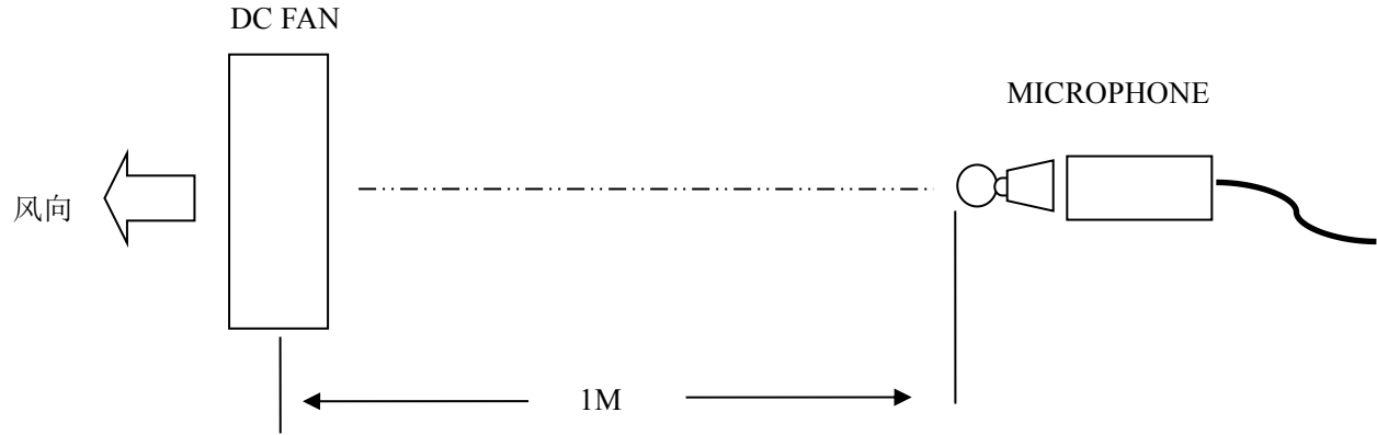
8-1.噪音测试方法示意图（Schematic diagram of noise test method）：
